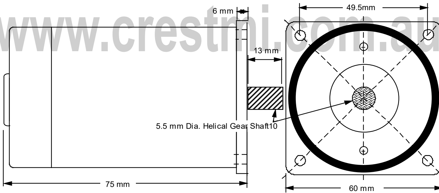
Precision DC PM Motor - Z2D10-12GN & Z2D10-24GN
