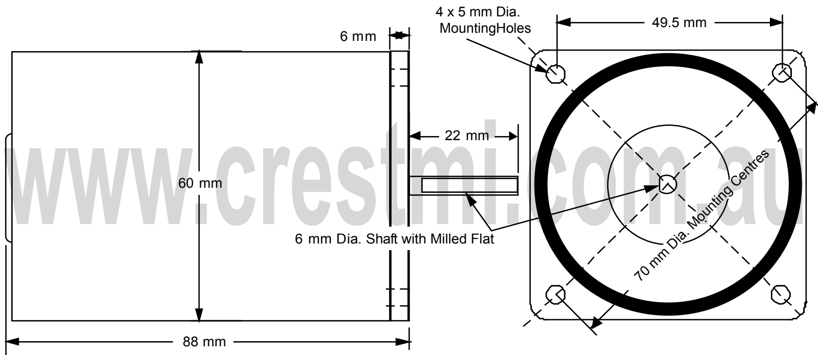
Precision DC PM Motor - Z2D10-12A & Z2D10-24A
